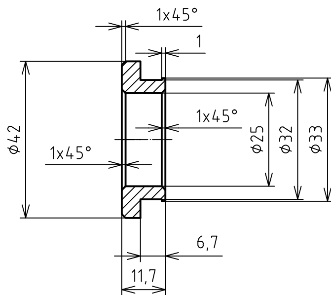
Rozpěrka 2ks
